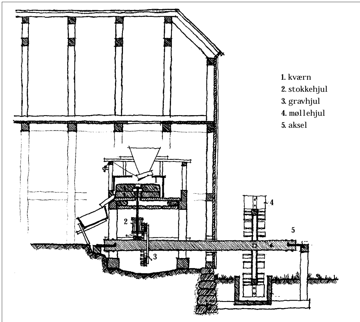
Rekonstruktions- tegnning af middel- alderlig vandmølle. Silkeborg Museum
