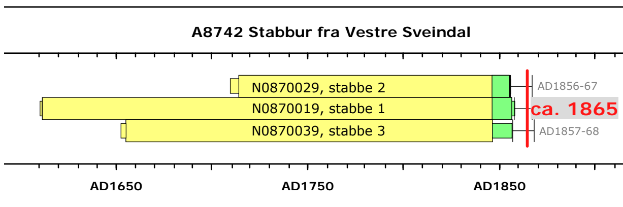
Figur 1: Dateringsdiagram. Stabber fra stabbur fra Vestre Sveindal, Audnedal kommune. Indplacering af de daterede prøver på en tidsskala. (Den grønne signatur angiver bevaret splintved.)
