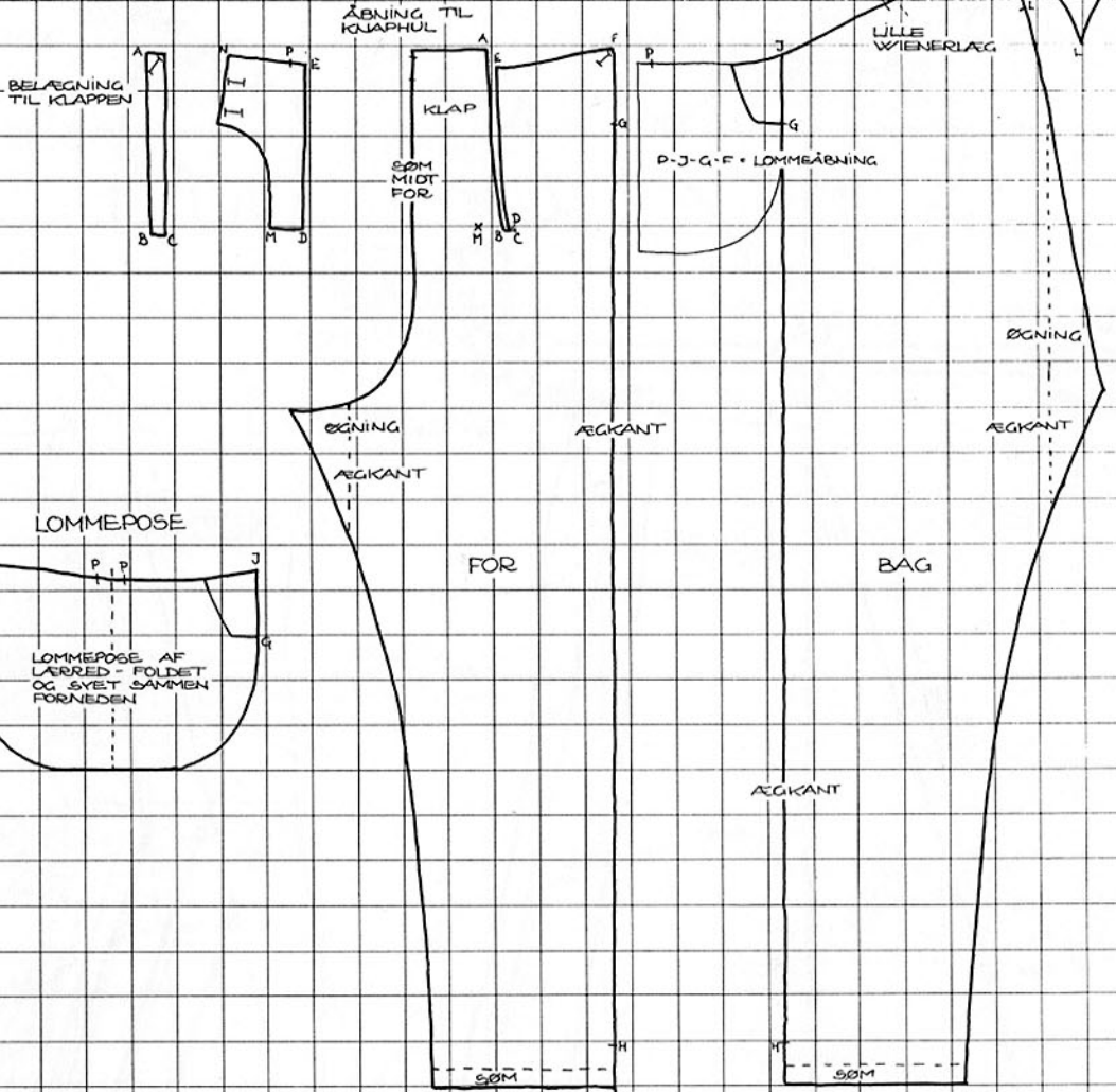
VENSTRE GAMACHE
