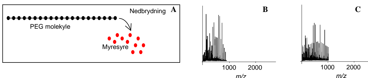
Fig. 2. A: Illustration som viser et PEG molekyle (sort) under nedbrydning til myresyre (rød). B: Massespektrum af PEG fra en Vasa prøve, de to PEG typer (600 og 1500) er rimeligt skarpt adskilte, det ser sundt ud. C: Massespektrum af PEG fra en anden Vasa prøve, de to PEG typer er mere sammenflydende, det ligner fordelingen af nedbrudt PEG.
